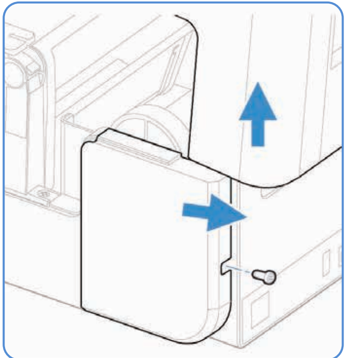
PC42E-T - Wi-Fi/BT Module Door
